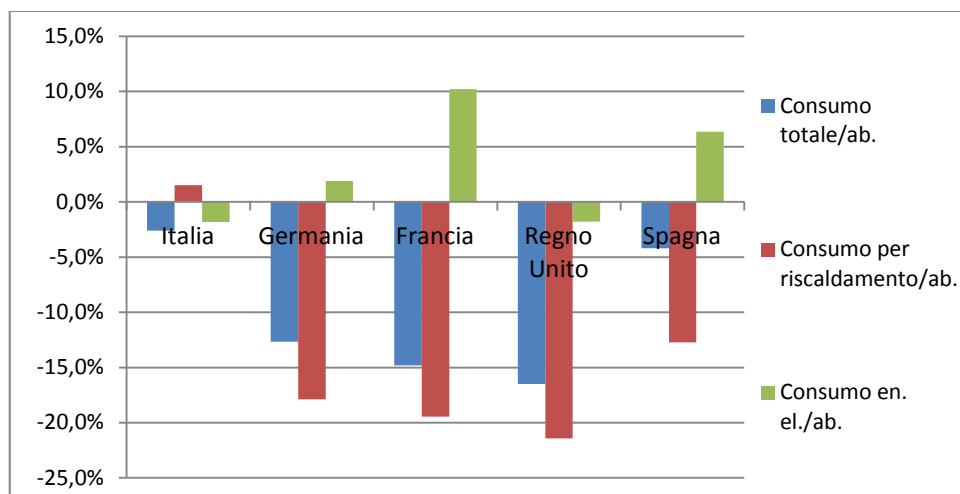
Figura 5: Variazione consumo totale, elettrico e del riscaldamento, per abitazione nel periodo 2000-2009 (Fonte: elaborazione ENEA su dati Odysee).
